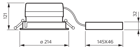
DN571B LED12S/830 PSED-E C WH
